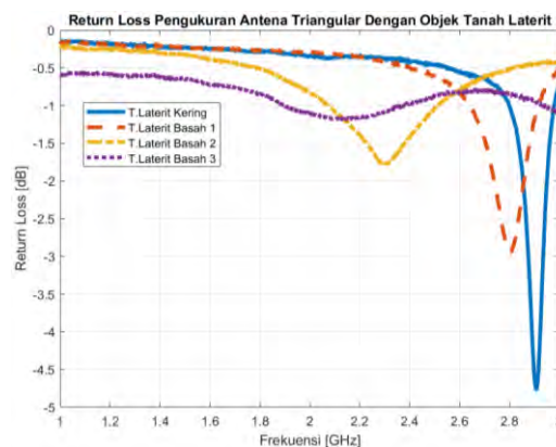
Gambar 14. Return Loss Antena Triangular Pada Tanah Laterit
