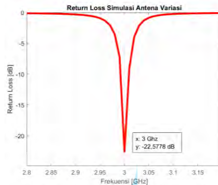
Gambar 8. Return Loss Simulasi Antena Variasi
