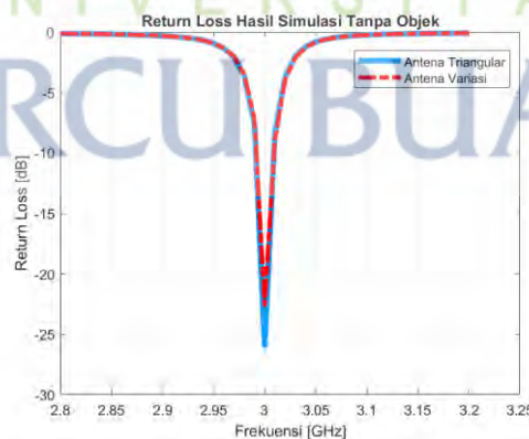
Gambar 9. Return Loss Simulasi Tanpa Objek
