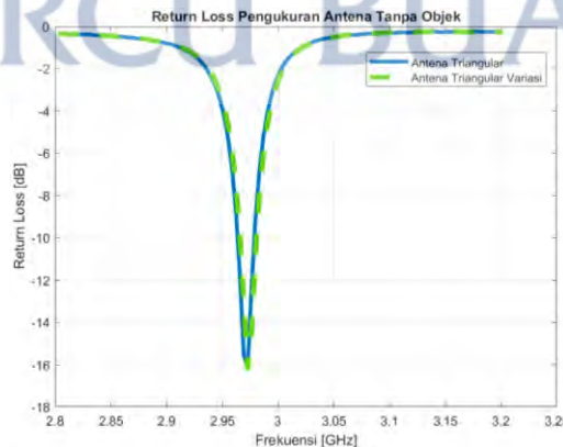
Gambar 11. Return Loss Pengukuran Tanpa Objek
