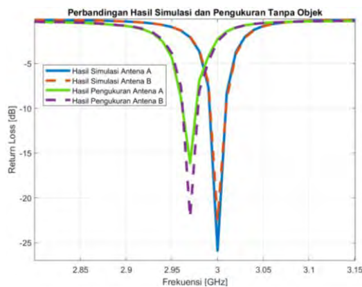
Gambar 16. Perbandingan Hasil Simulasi dan Pengukuran Tanpa Objek
