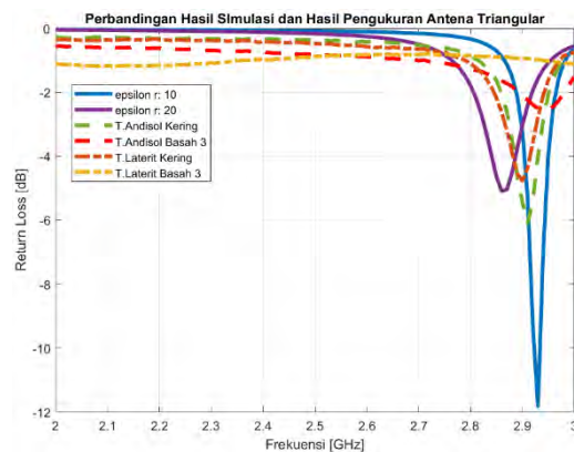
Gambar 17. Perbandingan Simulasi dan Pengukuran Objek Antena Triangular
