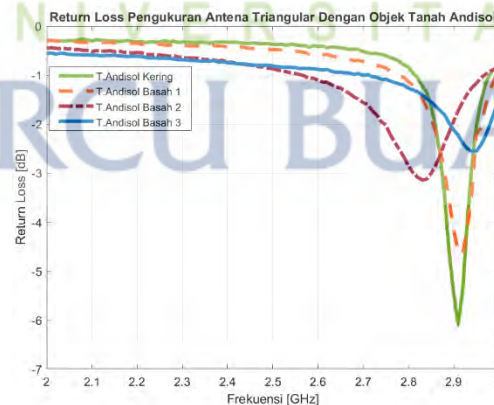
Gambar 12. Return Loss Antena Triangular Pada Tanah Andisol
