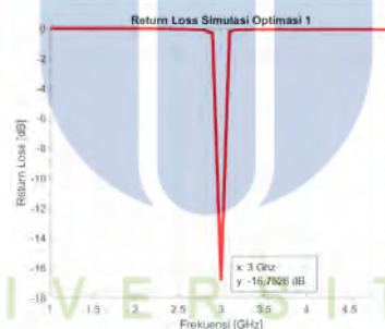
Gambar 4. Return Loss Hasil Optimasi Substrat dan Patch
