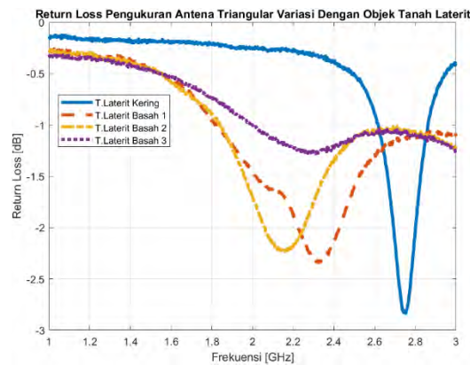
Gambar 15. Return Loss Antena Triangular Variasi Pada Tanah Laterit
