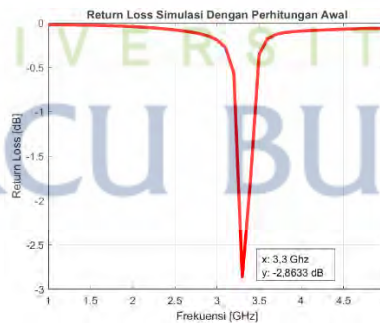
Gambar 3. Return Loss Simulasi Antena berdasarkan Perhitungan Awal
