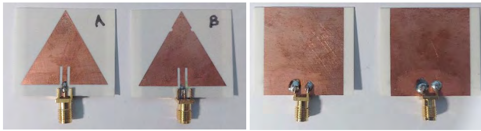
Gambar 10. Fabrikasi Antena Tampak Depan dan Tampak Belakang
