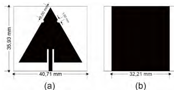
Gambar 7. Antena Variasi Patch (a) Tampilan Depan (b) Tampilan Belakang
