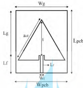
Gambar 2. Hasil Perancangan Antena Mikrostrip
