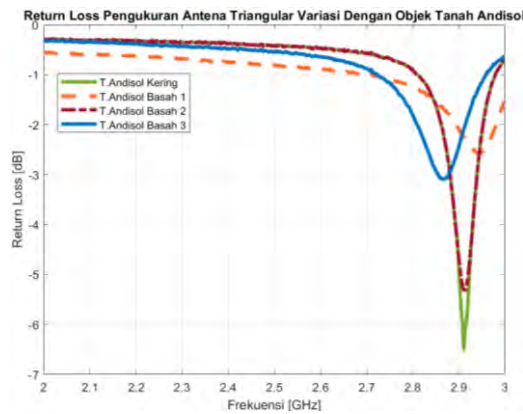
Gambar 13. Return Loss Antena Triangular Variasi Pada Tanah Andisol
