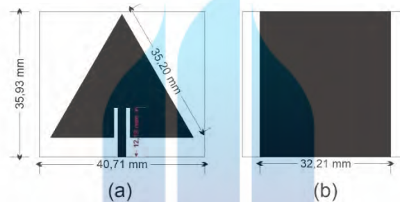
Gambar 6. Dimensi Antena (a) Tampilan Depan (b) Tampilan Belakang
