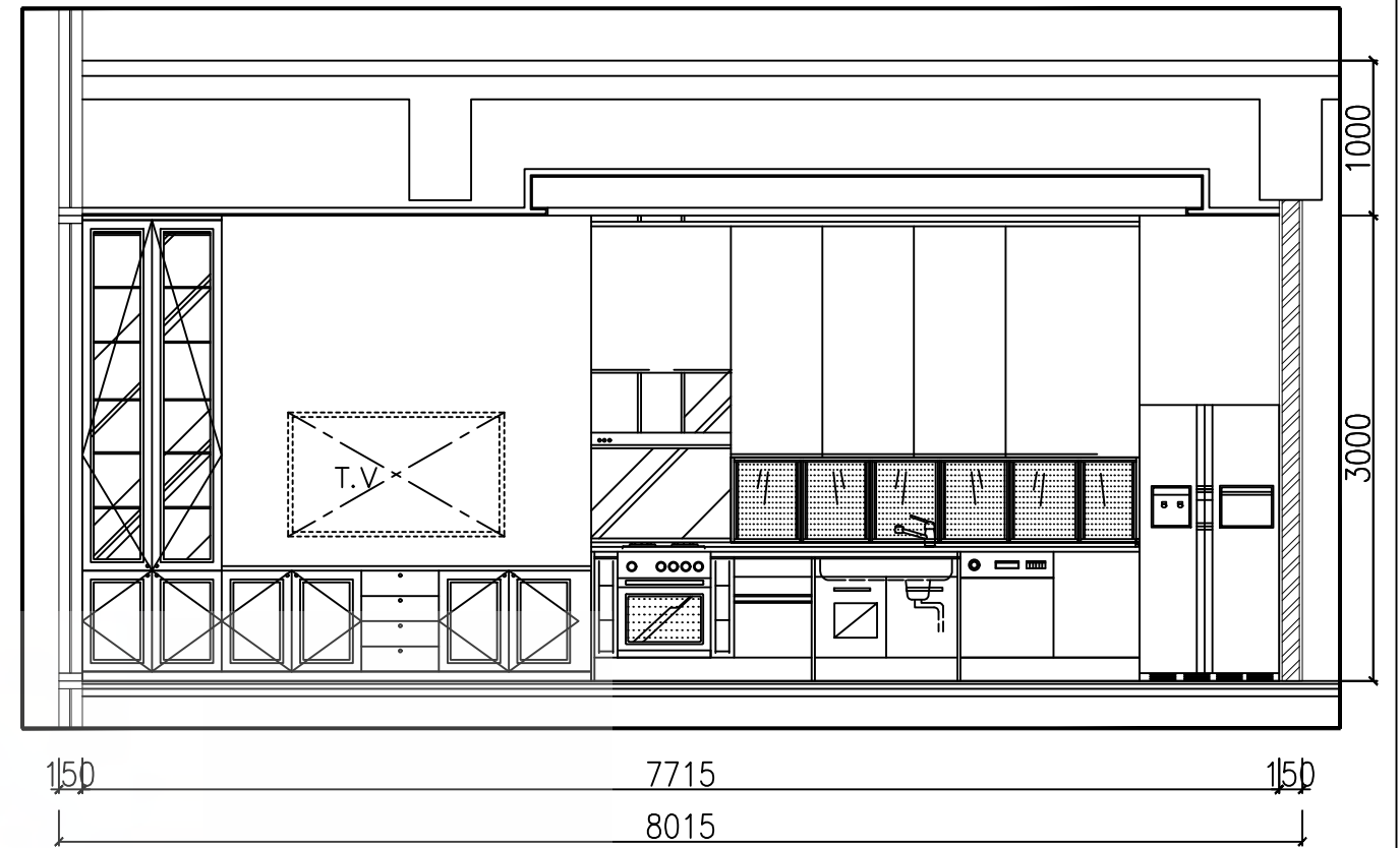
POTONGAN 1-1 SKALA 1 : 20
