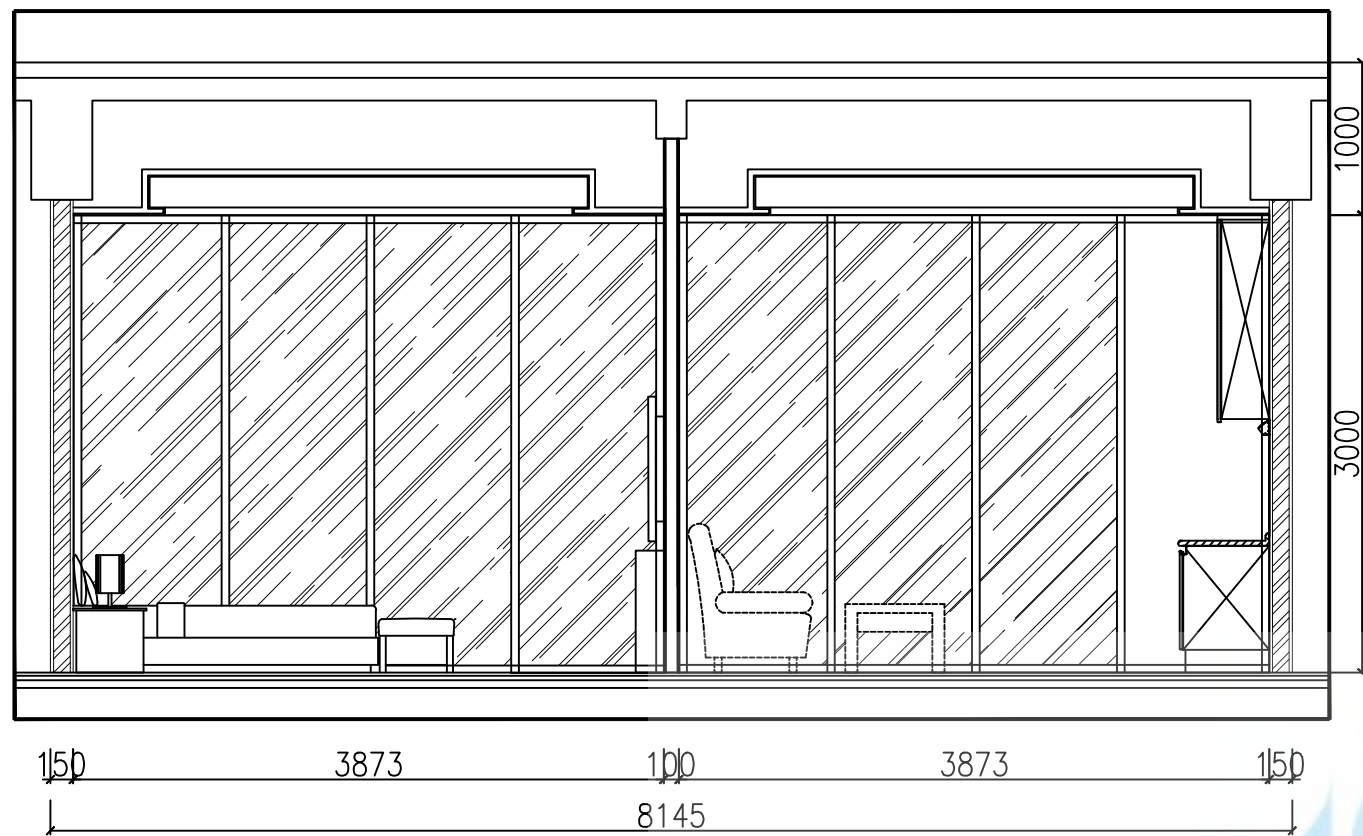
POTONGAN A-A SKALA 1 : 20
