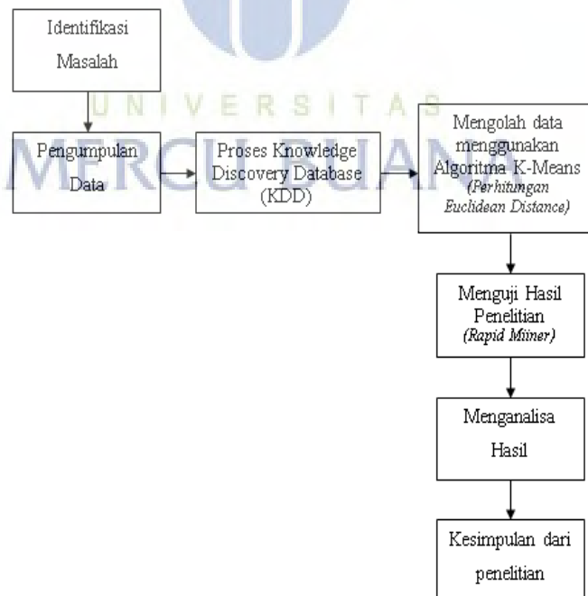
Gambar 2. Tahap Penelitian[5]
