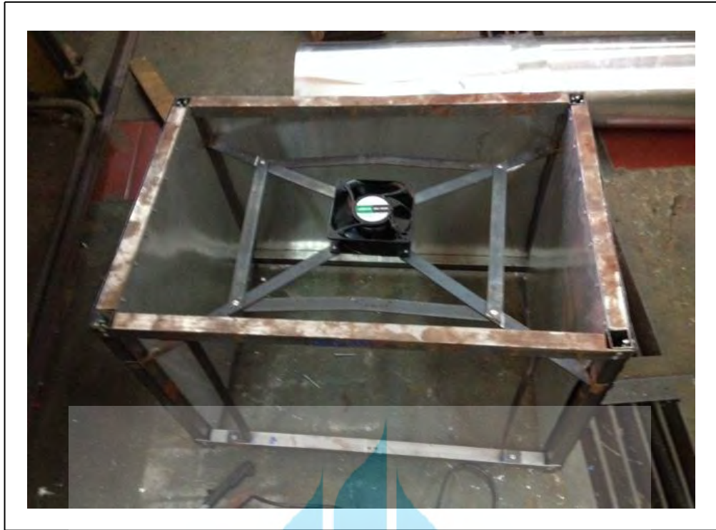
Penempatan Exhaust
