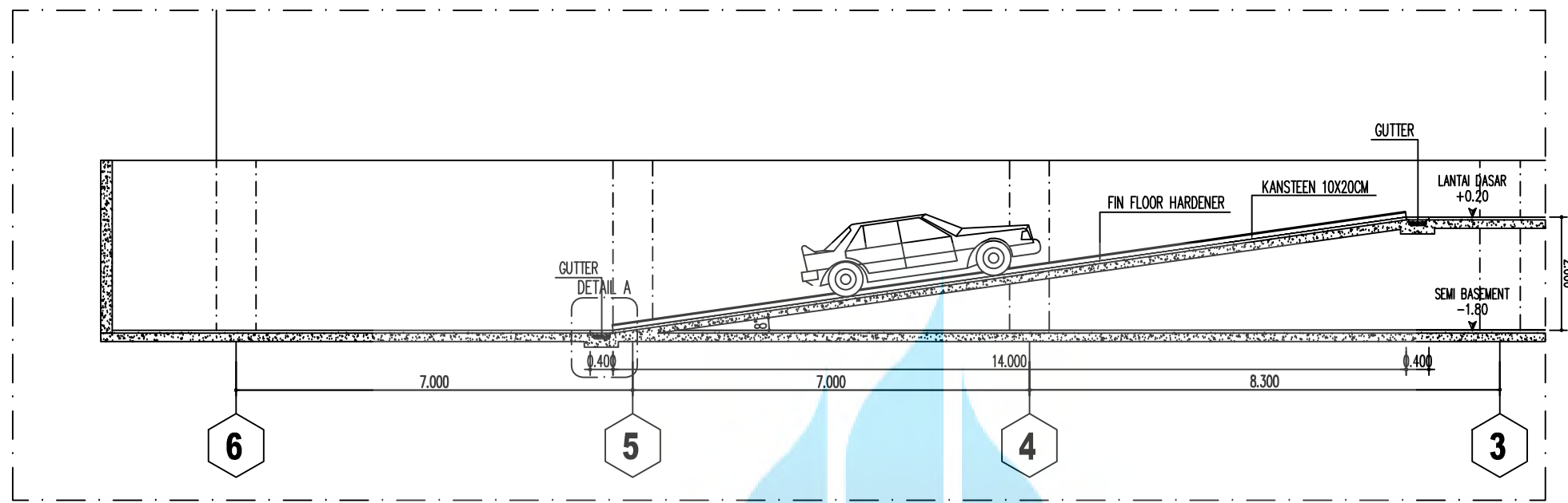
POTONGAN A.A SKALA 1 : 50
