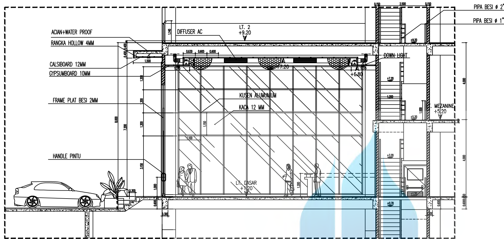
01 POTONGAN A-A' SKALA : 1 : 100
