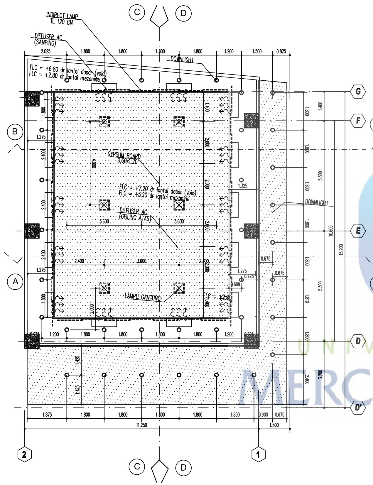
01 RENCANA POLA PLAFOND SKALA : 1 : 100
