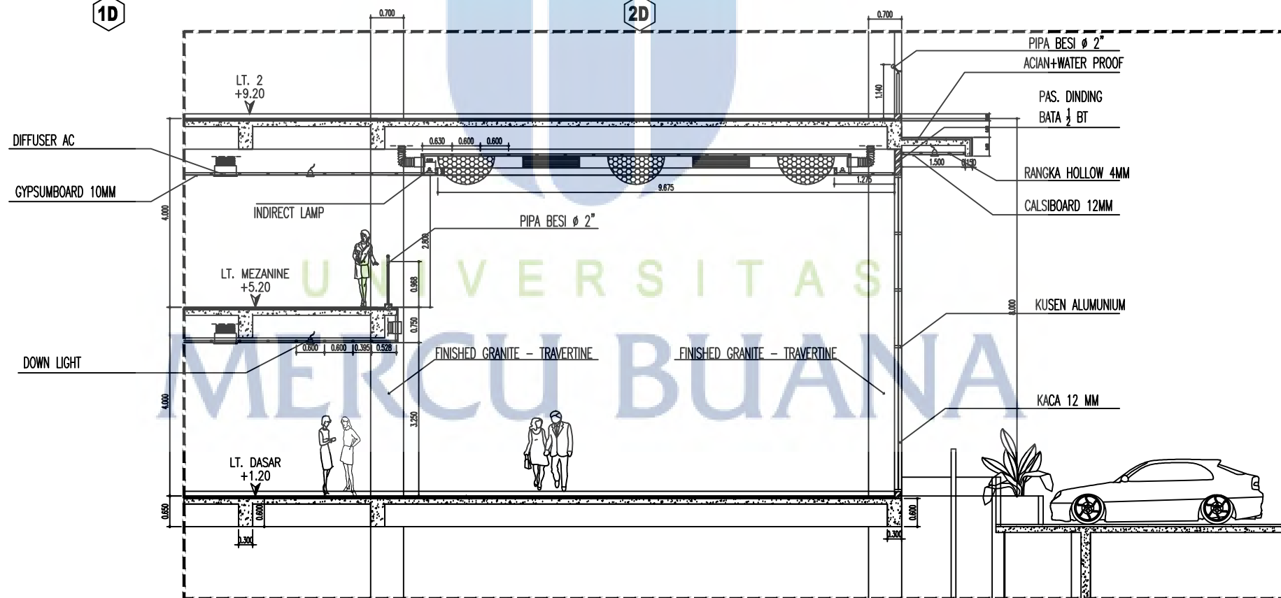
01 POTONGAN B-B' SKALA : 1 : 100
