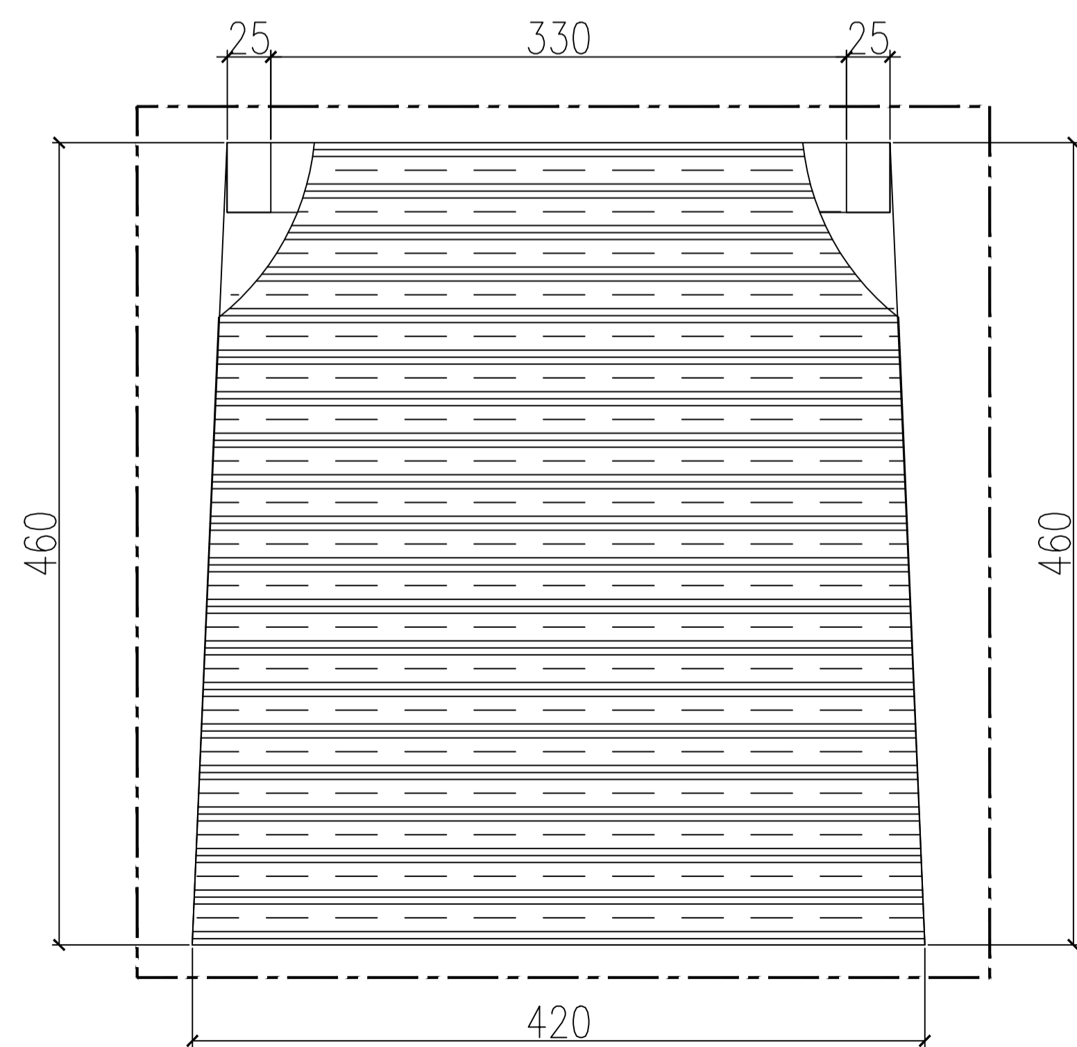
11 ID-GHB.11.2 TAMPAK ATAS KURSI SCALE 1:3
