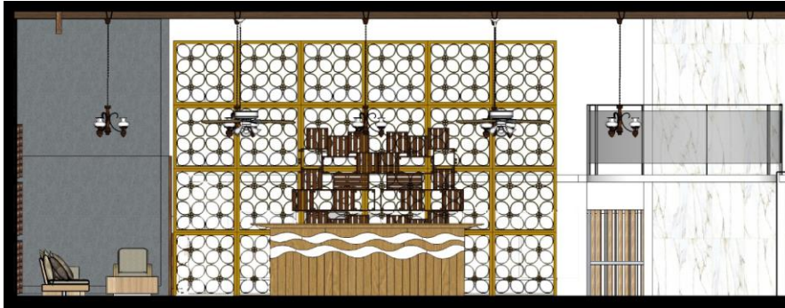
Tampak Potongan C-C Resepsionis Area
