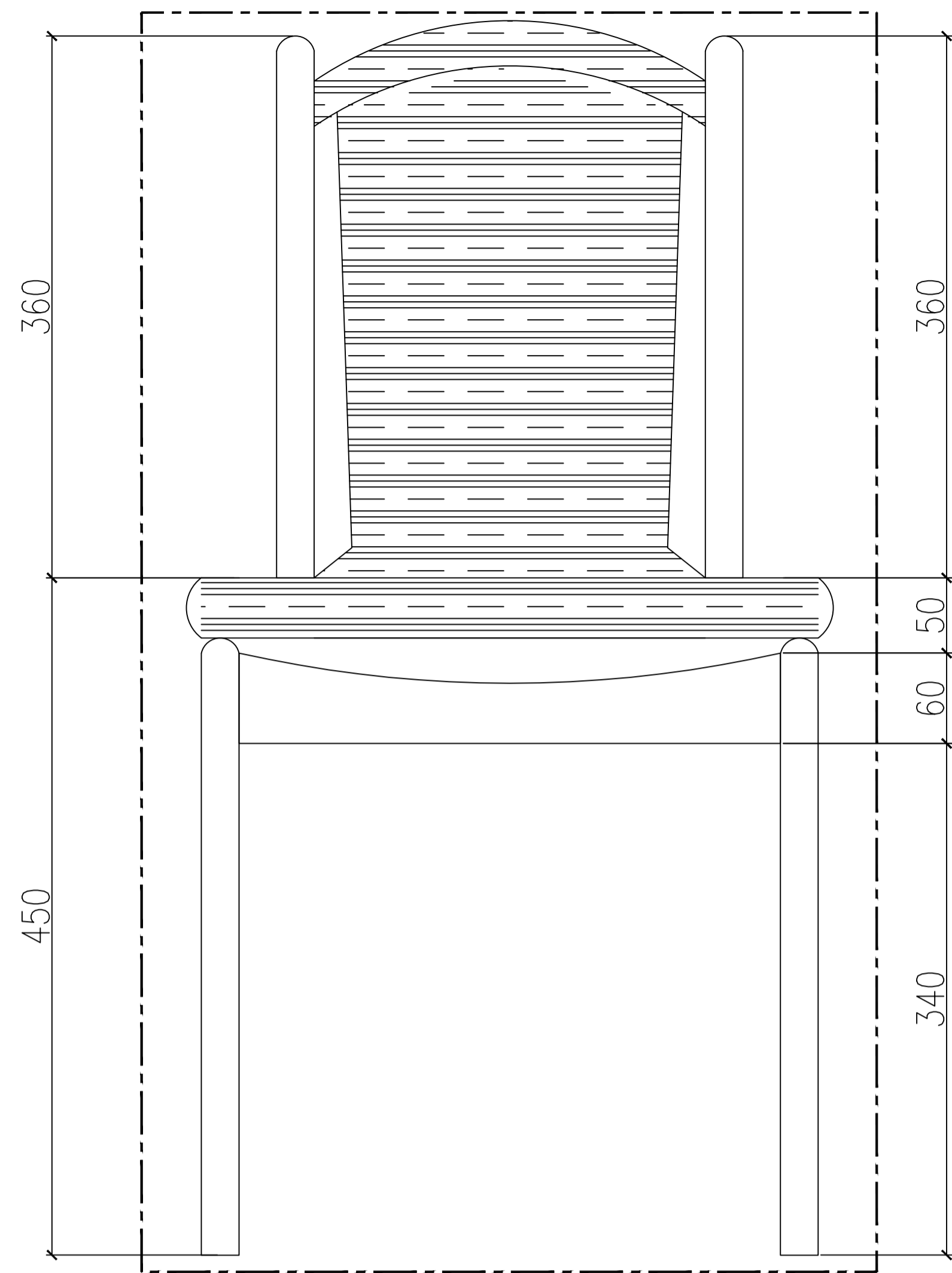
11 ID-GHB.11.0 TAMPAK DEPAN KURSI SCALE 1:3
