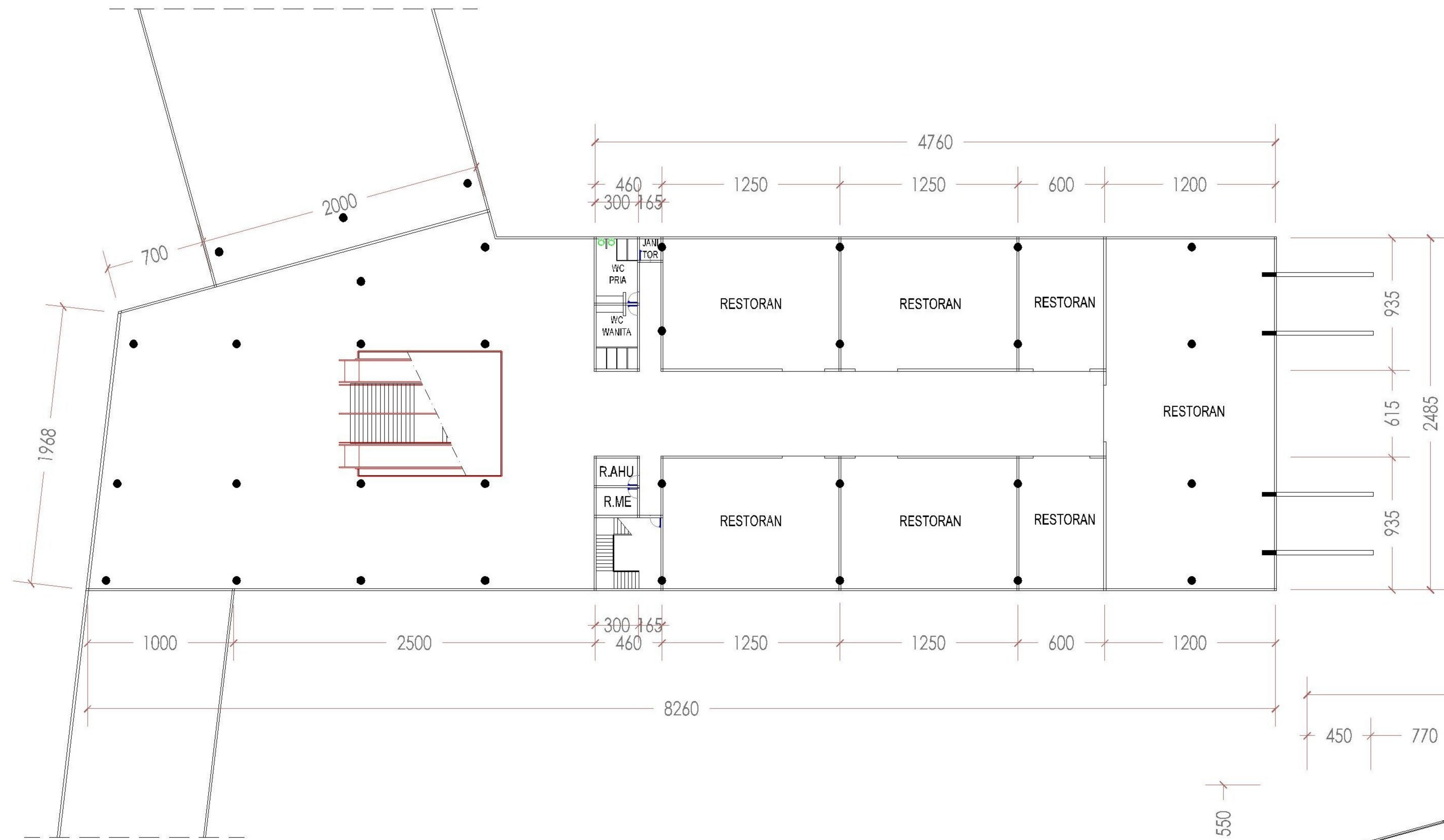
DENAH FASILITAS PENGHUBUNG LT.2
