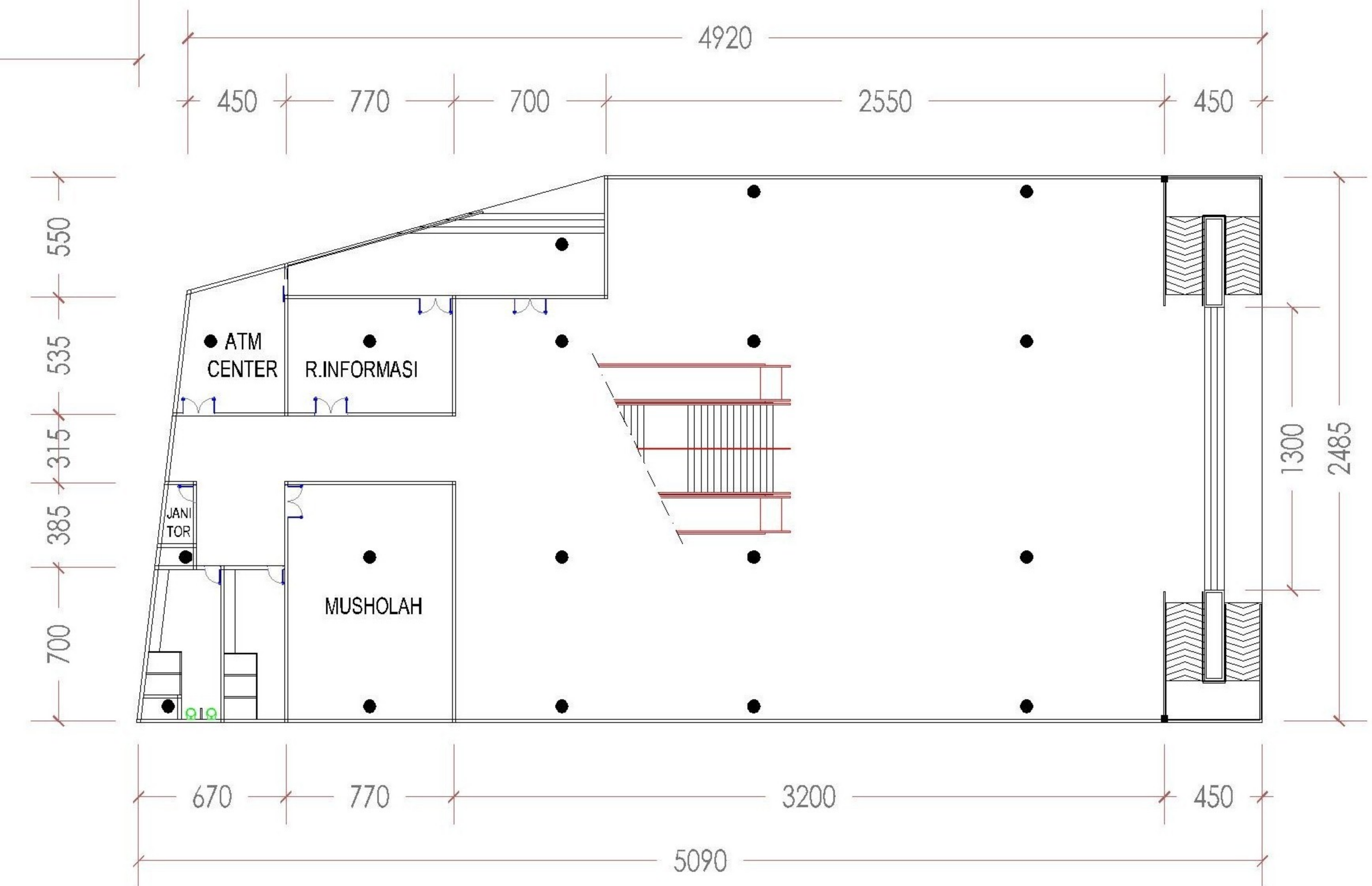
DENAH FASILITAS PENGHUBUNG LT.1
